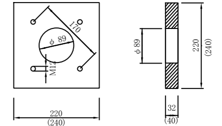
支圧板 S=1/5 (溶融亜鉛メッキ) (E5-4タイプ)
