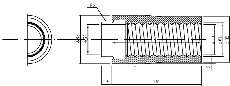
スペーサー S=1/1 #60
