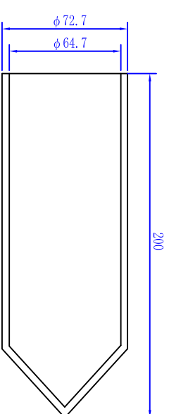
パイロットキヤッツフ 4型 S=1/3 φ72.7/64.7×200
