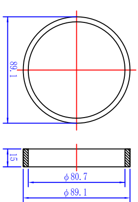
スチールリング 4型 S=1/3 φ89.1×15
