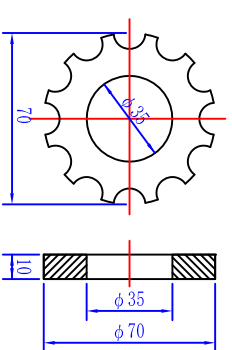
スチールリング 2型 S=1/3 φ70×10
