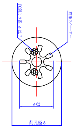
B-B断面図 S=1/3
