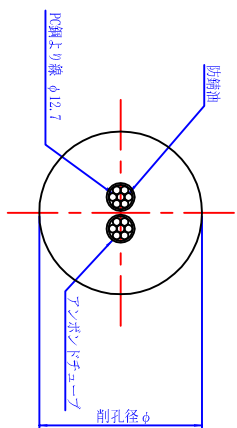
A-A断面図 S=1/3
